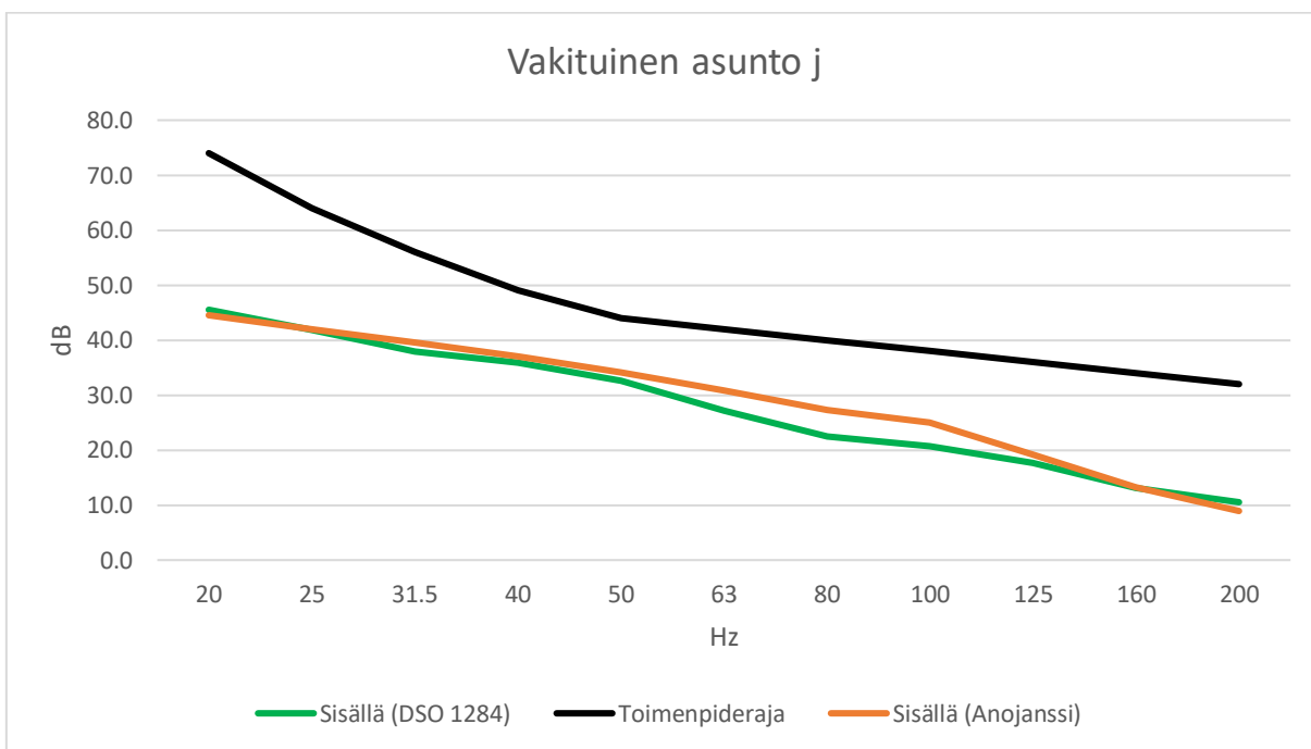
Kuva 2. Ympäristöministeriön ohjeistuksen mukainen pienitaajuisen melun laskenta sekä sosiaali- ja terveysministeriön toimenpiderajat vakituuisessa asunnossa j.
