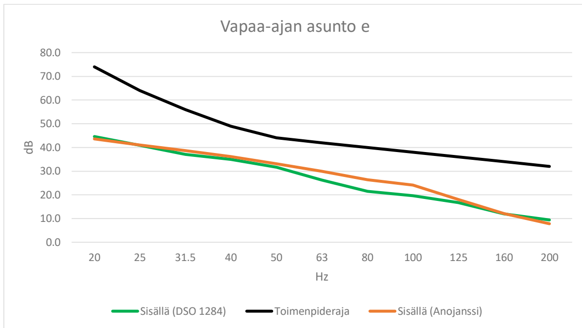
Kuva 3. Ympäristöministeriön ohjeistuksen mukainen pienitaajuisen melun laskenta sekä sosiaali- ja terveystieteiden ministeriön toimenpiderajat vapaa-ajan asunnossa e.
