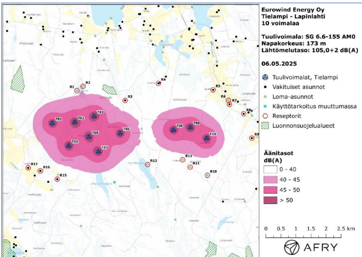
Kuva 42. Keskiäänitasot LAeq suunnittelualueella ja sen ympäristössä. © AFRY
