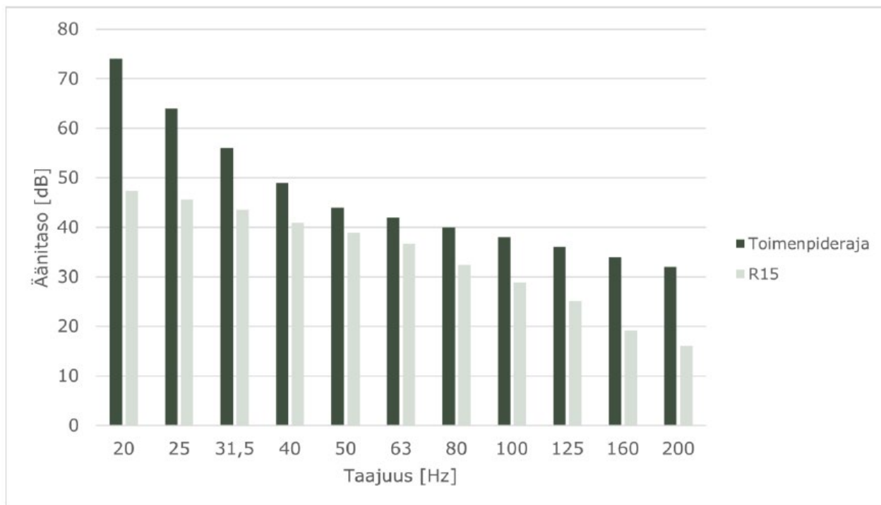
Kuva 72. Matalataajuisen sisämelun tasot reseptorin R15 kohdalla, kun mallinuksissa huomioidaan Tielammen ja Iso-Petäjämäen voimat. © AFRY
