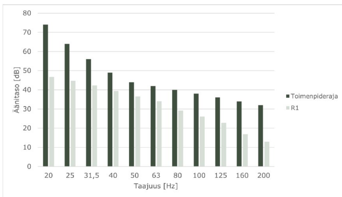
Kuva 43. Matalataajuisen sisämelun tasot verrattuna Asumisterveysasetuksen mukaisiin toimenpiderajoihin eri taajuuksilla reseptorin R1 kohdalla. © AFRY
