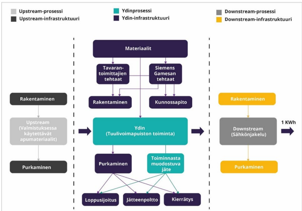
Kuva 64. Siemens Gamesa SG 6.6-155 EPD:n systeimirajat (Muokattu lähteestä: Muokattu lähteestä Siemens Gamesa – EPD (2022))
