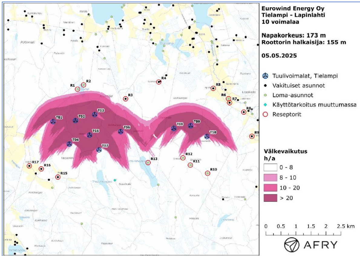
Kuva 44. Tuulivoimaloiden aiheuttama todennäköinen vuotuinen välkevaikutus ilman puuston vaikutusta. © AFRY
