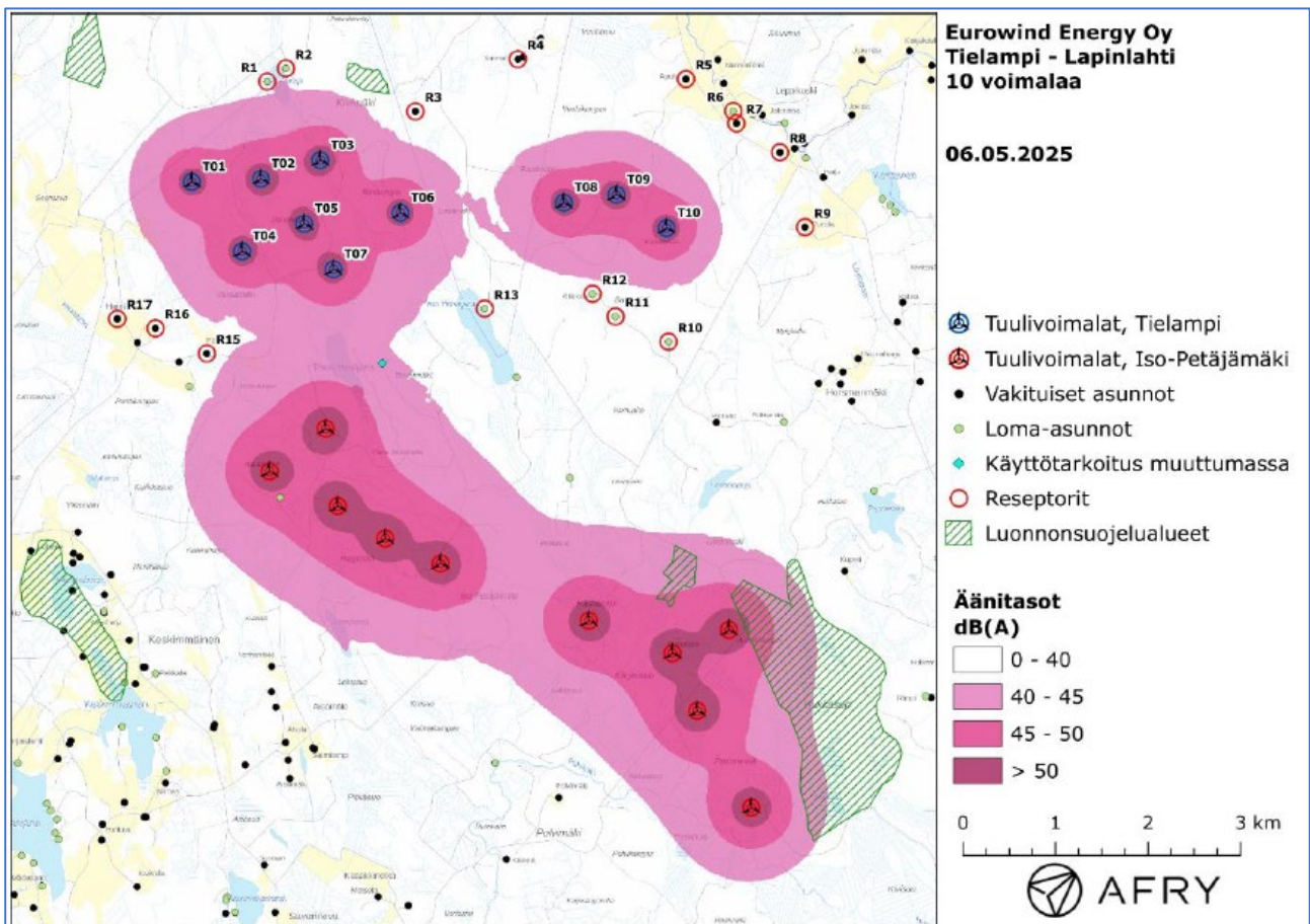
Kuva 71. Keskiäänitasot LAeq, kun mallinnuksissa huomioidaan Tielammen ja Iso-Petäjämäen voimalat. © AFRY
