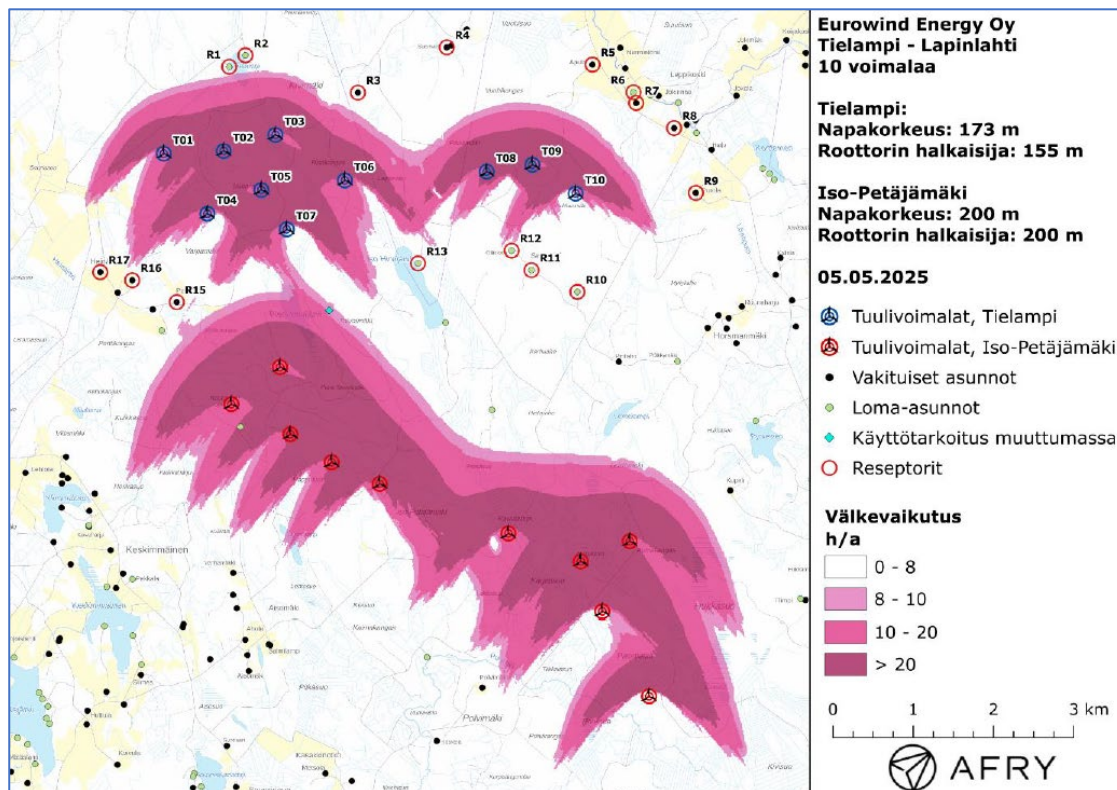
Kuva 73. Todennäköinen vuotuinen välkevaikutus, kun mallinnoissa huomioidaan Tielammen voimalat ja Iso-Petäjämäen voimalat, ilman puuston vaikutusta. © AFRY
