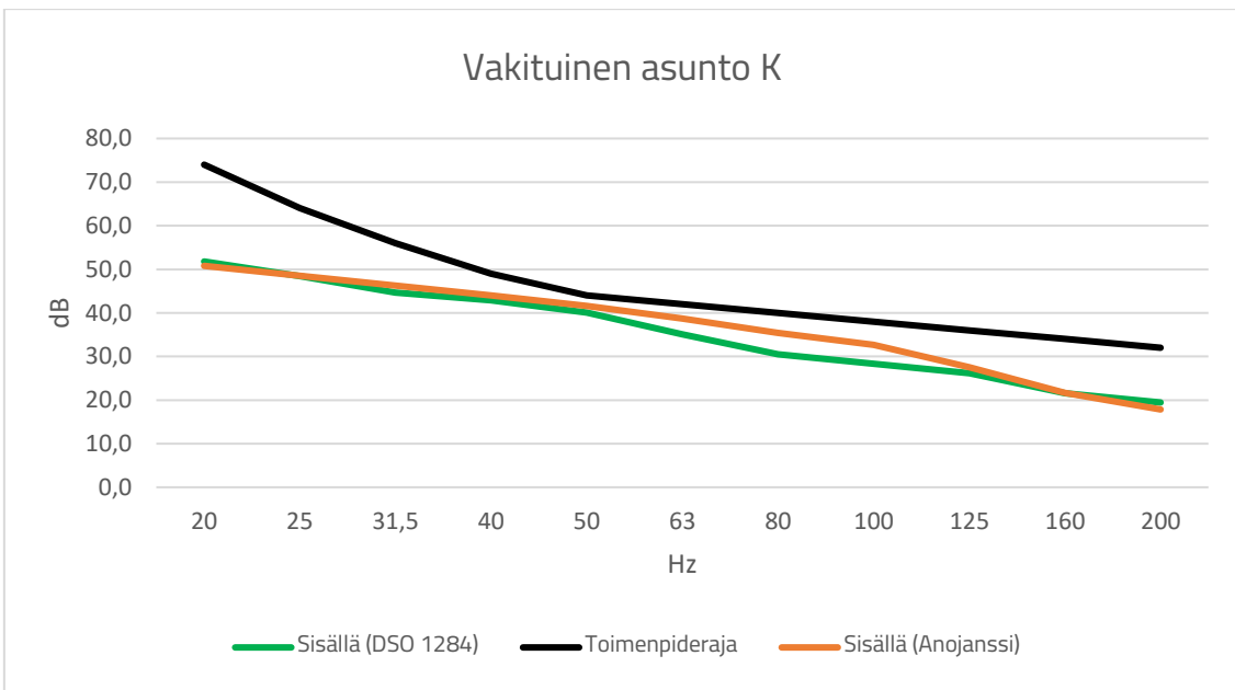
Kuva 9. Ympäristöministeriön ohjeistuksen mukainen pienitaajuisen melun laskenta sekä sosiaali- ja terveysministeriön toimenpiderajat vakituudessa asunnossa K.
