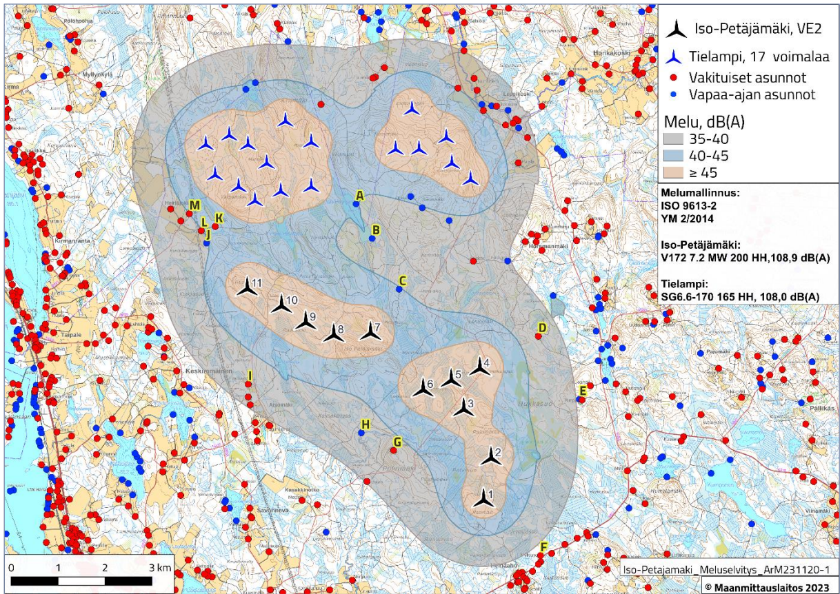
Kuva 4. Iso-Petäjämäen (VE2) ja naapuripuiston yhteisvaikutusten melumallinnus.
