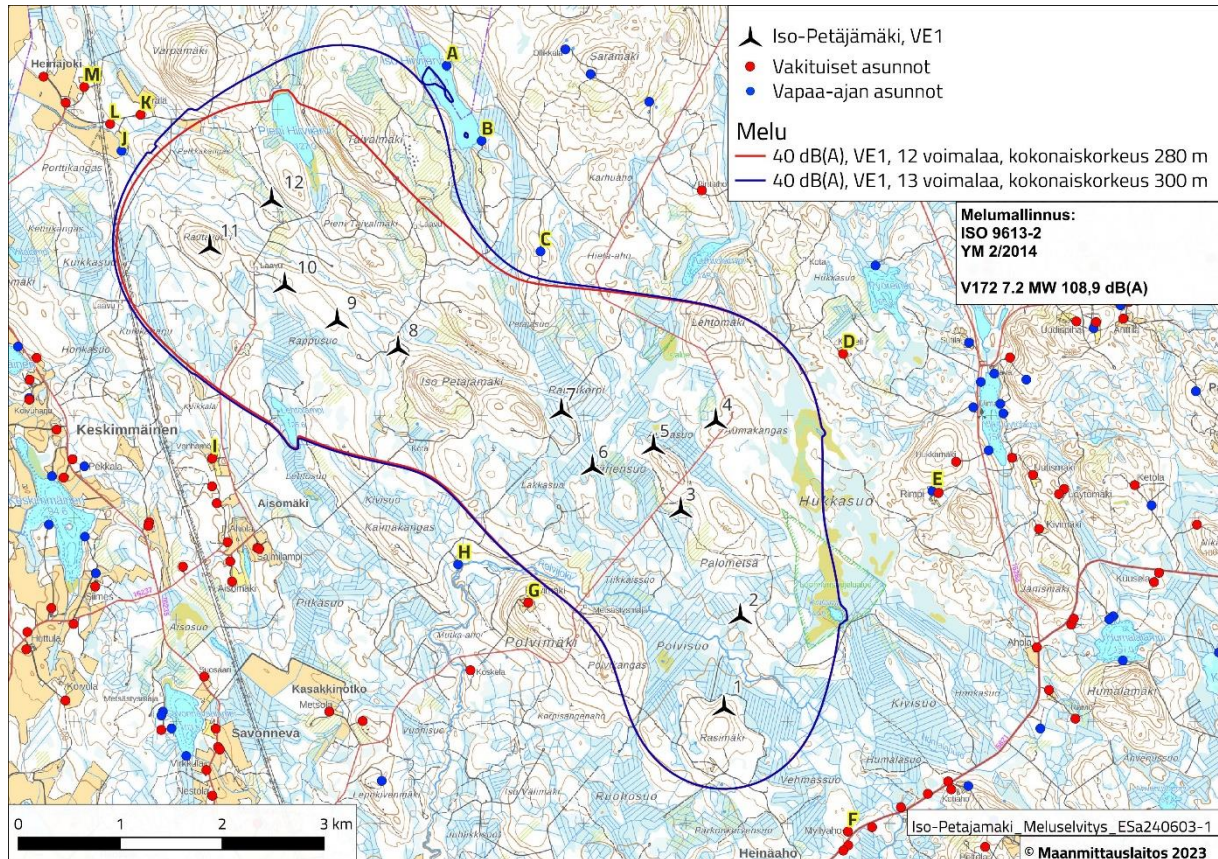
Kuva 13. Iso-Petäjämäen tuulivoimapuiston melumallinnus. Kuvassa on esitetty rajat, joiden sisäpuolella ylitetään valtioneuvoston asetuksen ohjearvo 40 dB(A).
