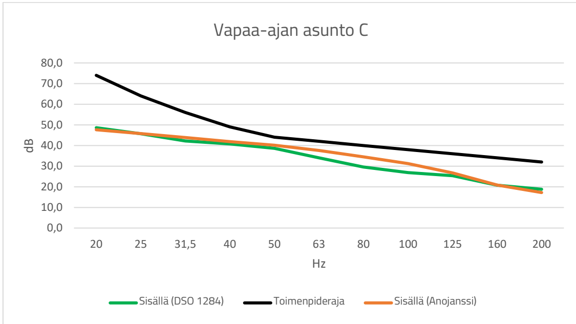
Kuva 10. Ympäristöministeriön ohjeistuksen mukainen pienitaajuisen melun laskenta sekä sosiaali- ja terveysministeriön toimenpiderajat vapaa-ajan asunnossa C.
