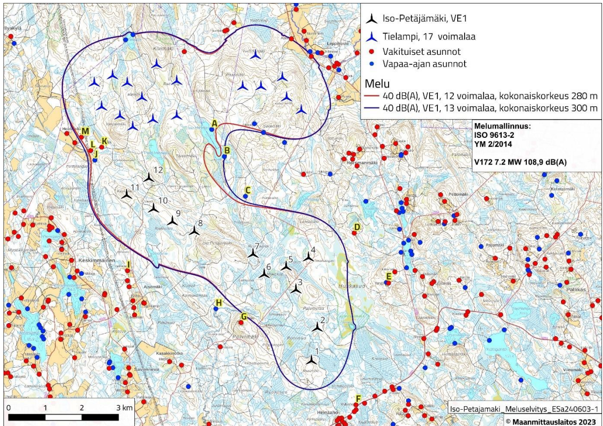
Kuva 14. Iso-Petäjämäen (VE1) ja naapuripuiston yhteisvaikutusten melumallinnus. Kuvassa on esitetty rajat, joiden sisäpuolella ylitetään valtioneuvoston asetuksen ohjearvo 40 dB(A).
