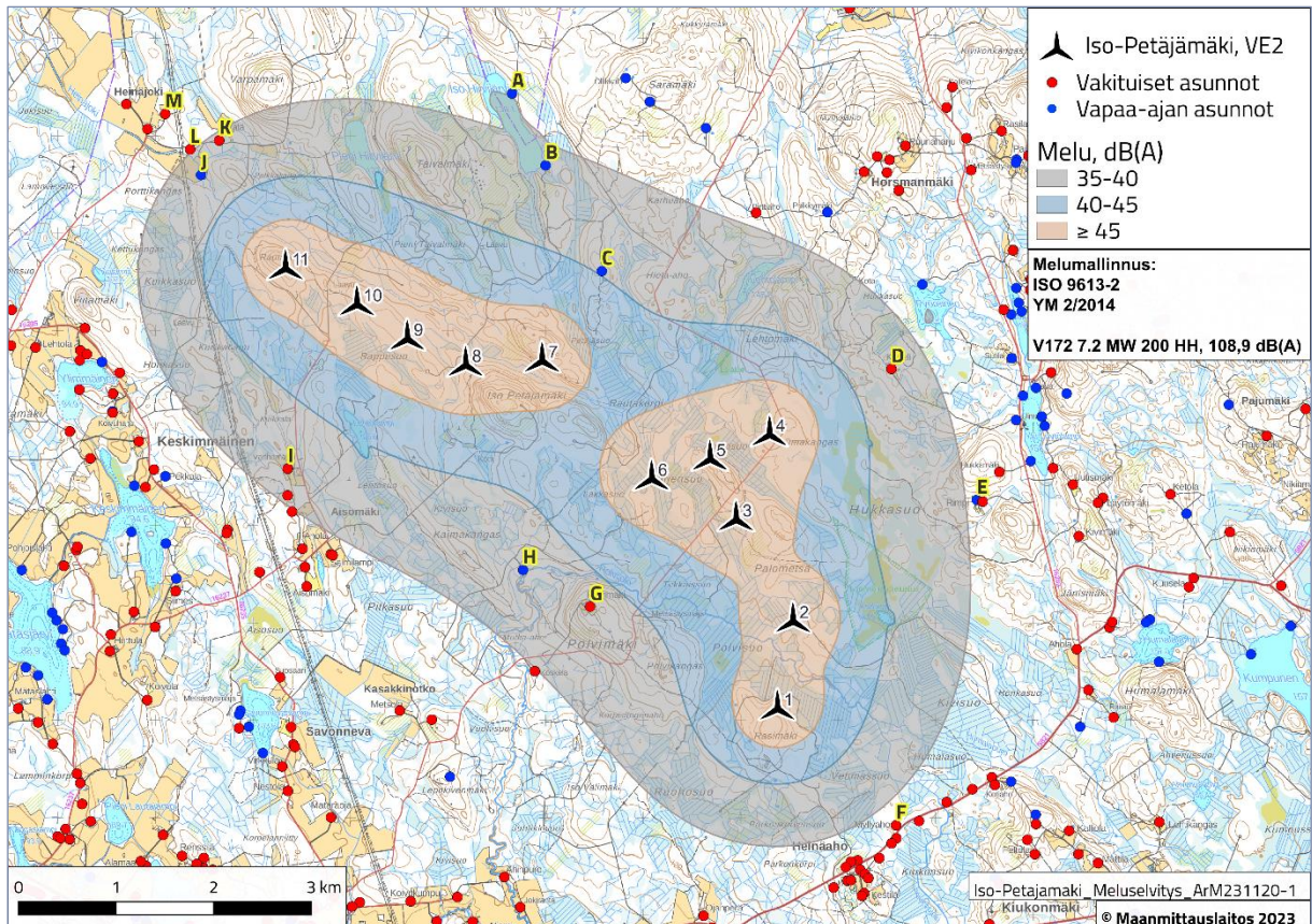
Kuva 2. Iso-Petäjämäen tuulivoimapaiston melumallinnus (VE2), V172 7.2 MW 200HH, 106,9 + 2 dB(A). 13 havainnointipistettä on merkitty kuvaan kirjaimilla.
