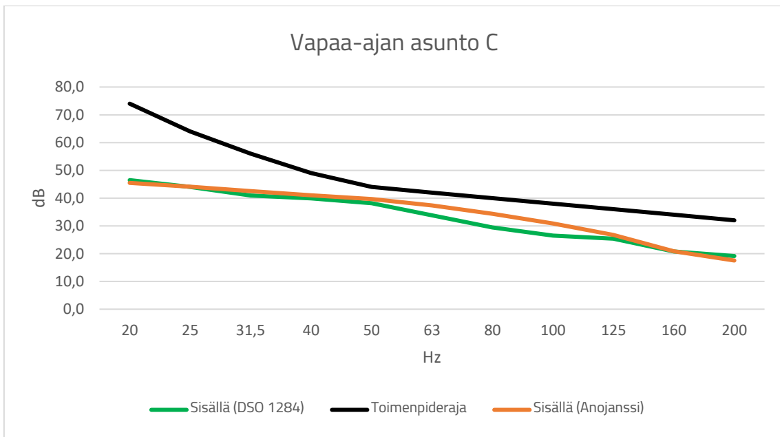
Kuva 8. Ympäristöministeriön ohjeistuksen mukainen pienitaajuisen melun laskenta sekä sosiaali- ja terveysministeriön toimenpiderajat vapaa-ajan asunnossa C.
