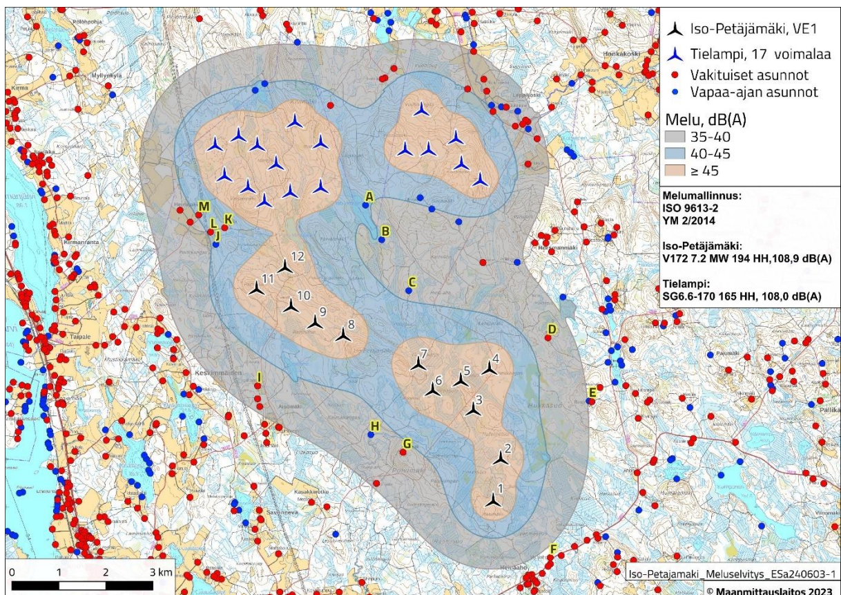
Kuva 3. Iso-Petäjämäen (VE1) ja naapuripuiston yhteisvaikutusten melumallinnus.
