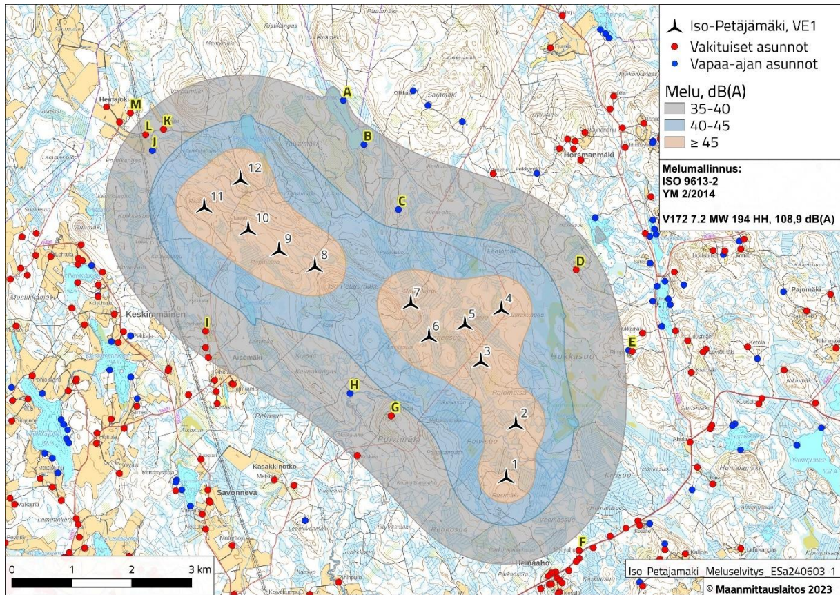
Kuva 1. Iso-Petajämäen tuulivoimapuiston melumallinnus (VE1), V172 7.2 MW 194 HH, 106,9 +2 dB(A). 13 havainnointipistettä on merkitty kuvaan kirjaimilla.
